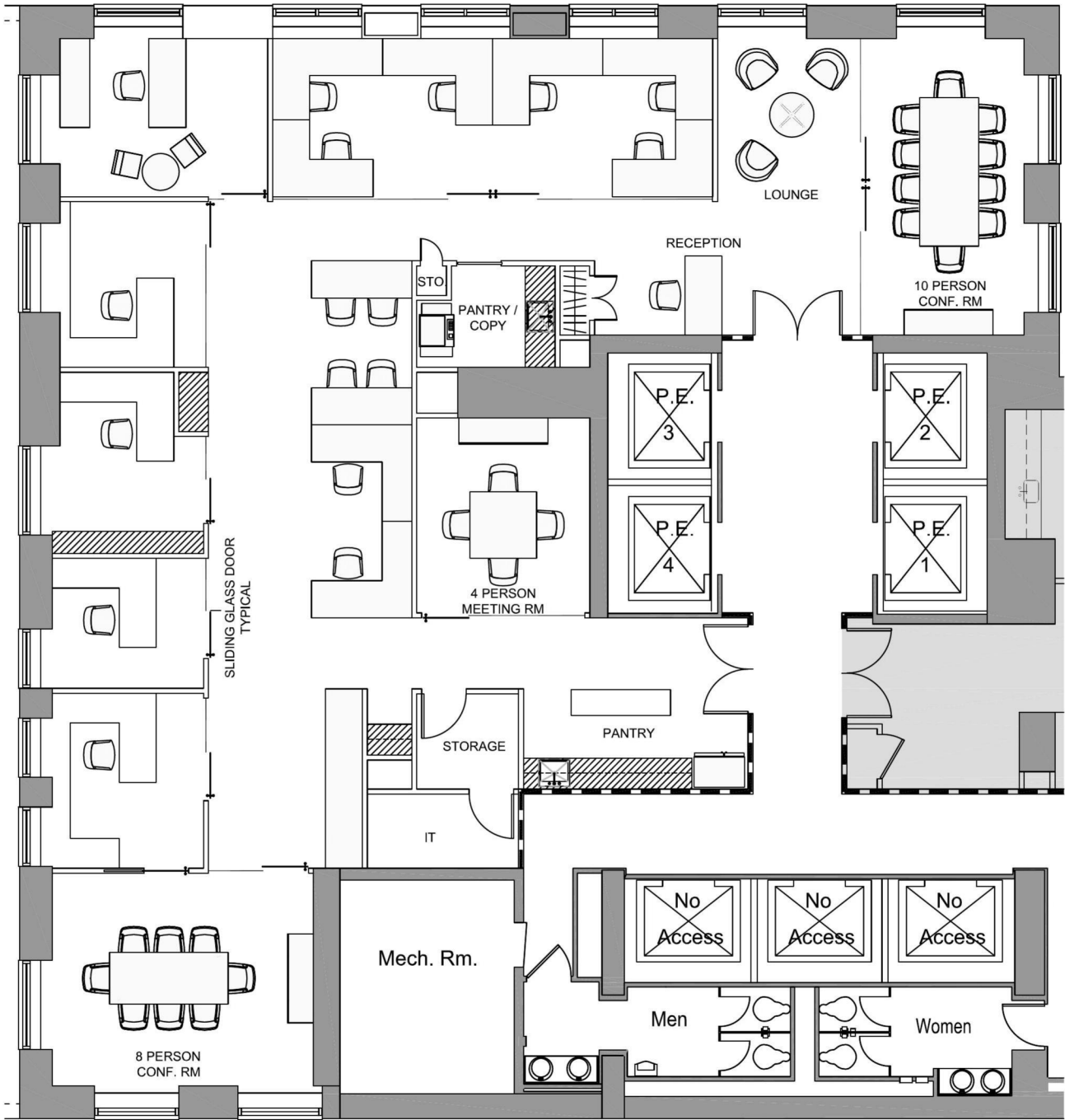
Scale: 3/32" = 1'-0"
